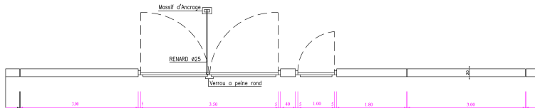
PORTE D'ENTREE VUE EN PLAN
