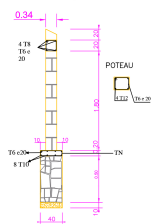
C O U P E A - A ECH : 1/50
