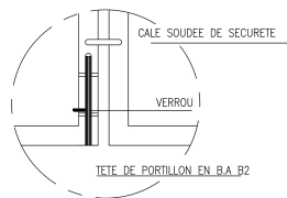
D E T A I L - B - PORTILLON
